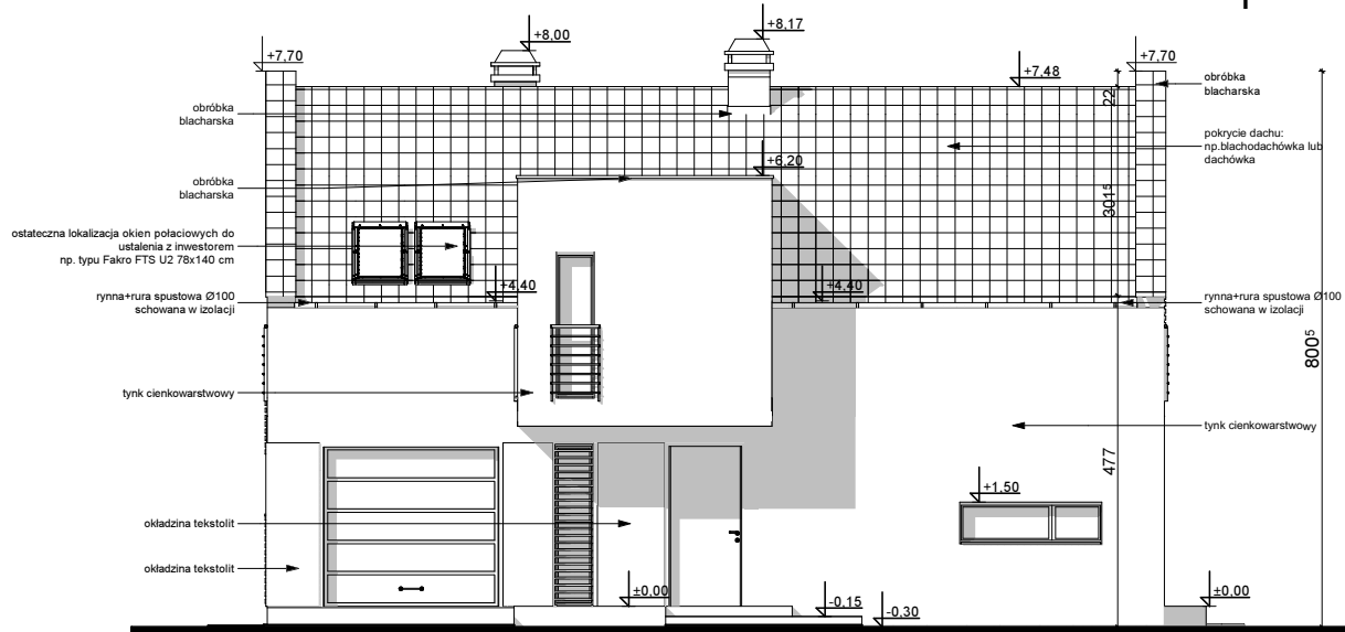
ELEWACJA FRONTOWA
