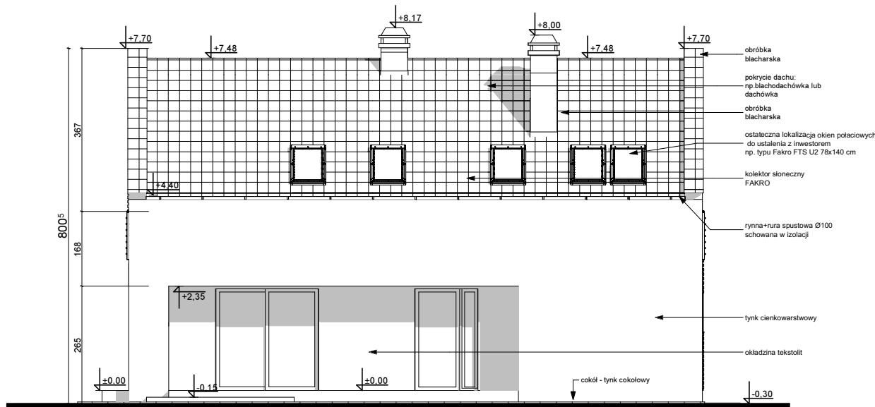
ELEWACJA OGRODOWA (tylna)
